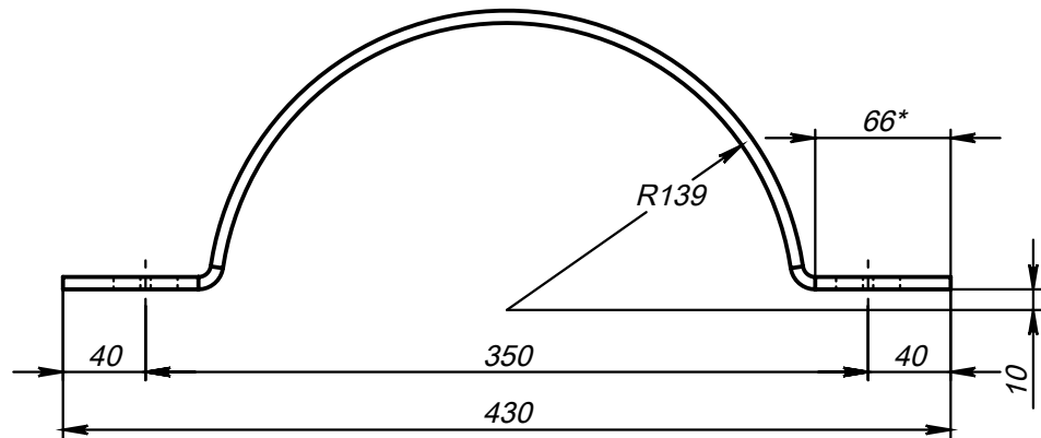
Поз.1 (Полухомут)
