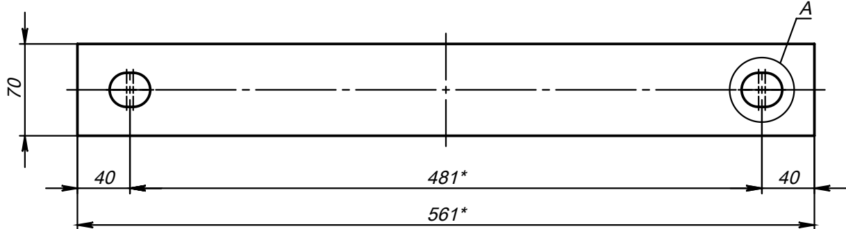
Поз.1 (Полухомут) развертка
